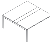
SY06 1600 / 1610 / 740 79.9 kg
