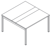
SY42 1200 / 1210 / 740 46.7 kg
