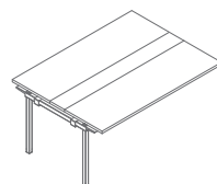
SY56 1600 / 1210 / 740 51.2 kg
